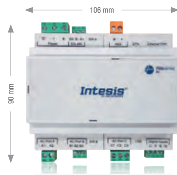
ME-AC-MBS-KNX-HA Schnittstelle
