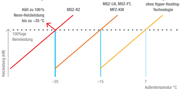
Verbesserte Heizleistung
