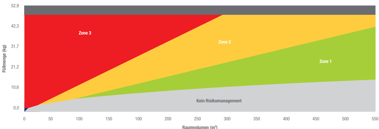
Bestimmung der Sicherheitszone
