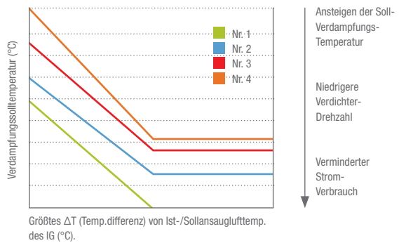
Energieeffiziente Verdampfungskontrolle
