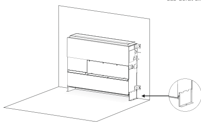
Bodenansaugung/Montage auf dem Boden stehend mit Füßen.
