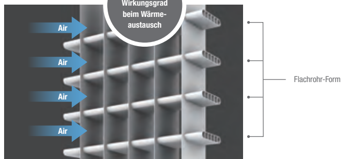
Flachrohr-Wärmetauscher
