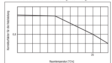
Abb. 4 Temperaturabhängige Korrektur der Innengeräte Nur für die Korrektur der Heizleistungen der Innengeräte
