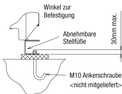
Bild B (mit montierten Stellfüßen)
