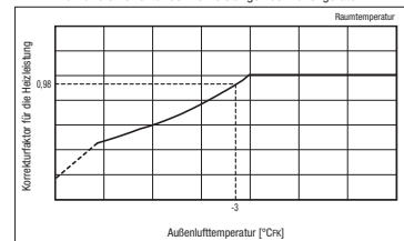
Abb. 5 Temperaturabhängige Korrektur der Außengeräte Nur für die Korrektur der Heizleistungen der Außengeräte
