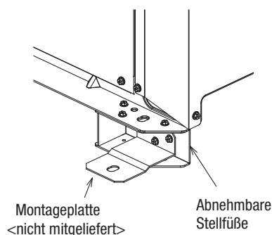
Bild D (mit montierten Stellfüßen)
