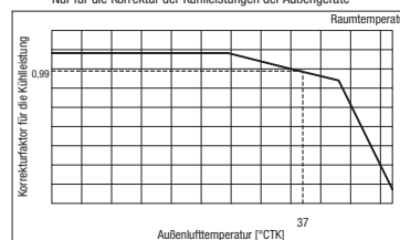
Abb. 2 Temperaturabhängige Korrektur der Außengeräte Nur für die Korrektur der Kühlleistungen der Außengeräte
