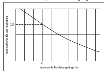
Abb. 6 Korrekturfaktor der äquivalenten Rohrleitungslänge
