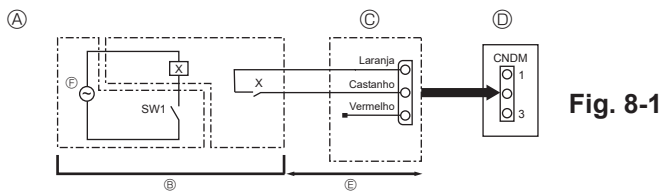
Fig. 8-1 A Exemplo de diagrama de circuito (modo de baixo nível de ruído) B Disposição no local C Adaptador de entrada externo (PAC-SC36NA-E) X: Relé D Painel de controle da unidade exterior E Máx. 10 m F Alimentação para relé
