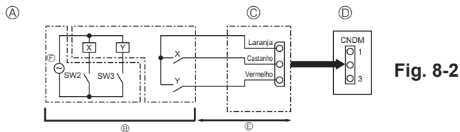
Fig. 8-2 A Exemplo de diagrama de circuito (Função de pedido) B Disposição no local X, Y: Relé C Adaptador de entrada externo (PAC-SC36NA-E) D Painel de controle da unidade exterior E Máx. 10 m F Alimentação para relé
