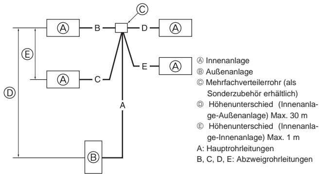
<Grenzen für Verlegung von Kältemittelrohrleitungen>
