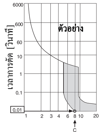
กราฟตัวอย่างการตัดกระแสไฟที่ระบุ (x) กราฟตัวอย่าง
