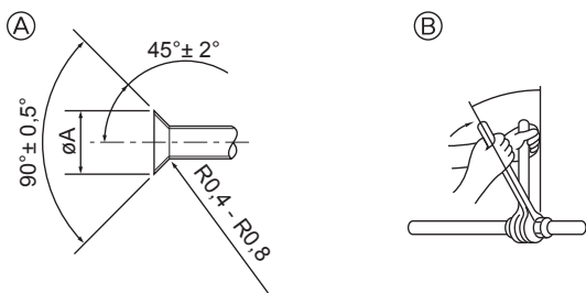
Ⓐ Abmessungen der Aufweitungsschnitte Ⓑ Anzugsdrehmoment für die Konusmutter
