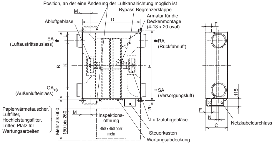
Lossnay-Papierwärmetauscher Befestigungsposition für Hochleistungsfilter (separat erhältlich)
