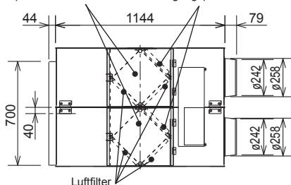
Lossnay-Papierwärmetauscher Befestigungsposition für Hochleistungsfilter (separat erhältlich)
