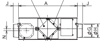
Lossnay-Papierwärmetauscher Befestigungsposition für Hochleistungsfilter (separat erhältlich)
