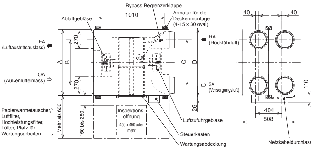
Lossnay-Papierwärmetauscher Befestigungsposition für Hochleistungsfilter (separat erhältlich)
