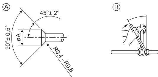
Ⓐ Abmessungen der Aufweitungsschnitte Ⓑ Anzugsdrehmoment für die Konusmutter
