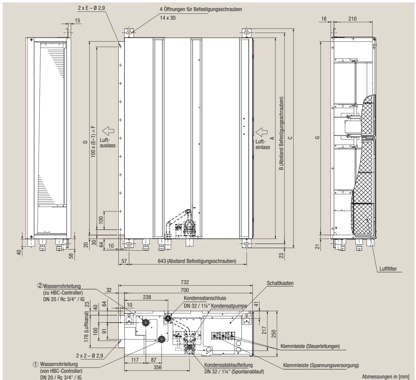
Abbildung 4.12 Abmessungen PEFY-WP20/25/32/40/50VMA-E
