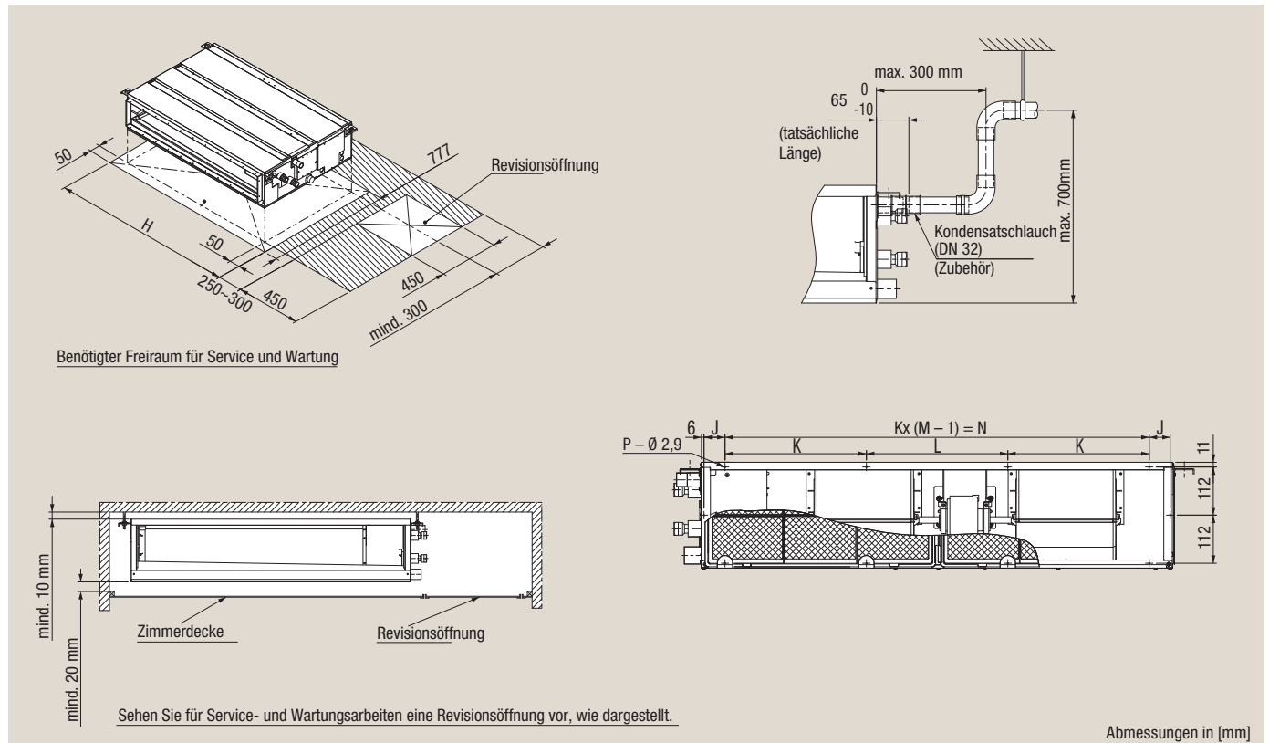
Abbildung 4.13 Installationsfreiraum PEFY-WP20/25/32/40/50VMA-E
