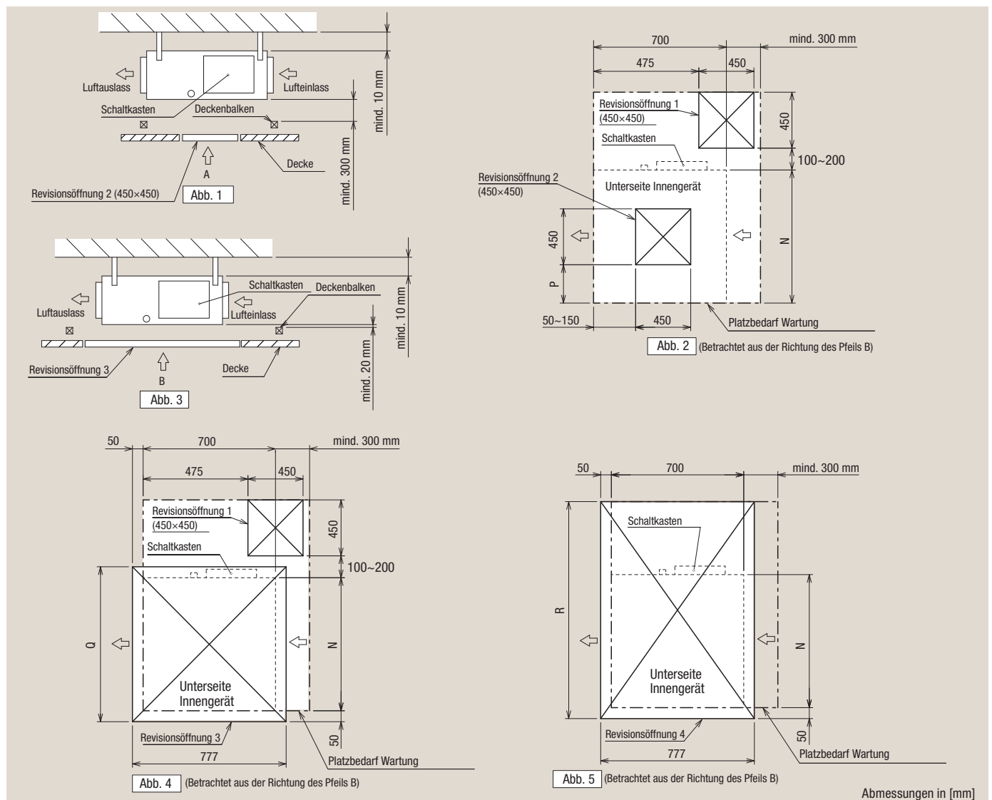
Abbildung 4.10 Installationsfreiraum PEFY-WP15/20/25/32/40/50VMS1-E
