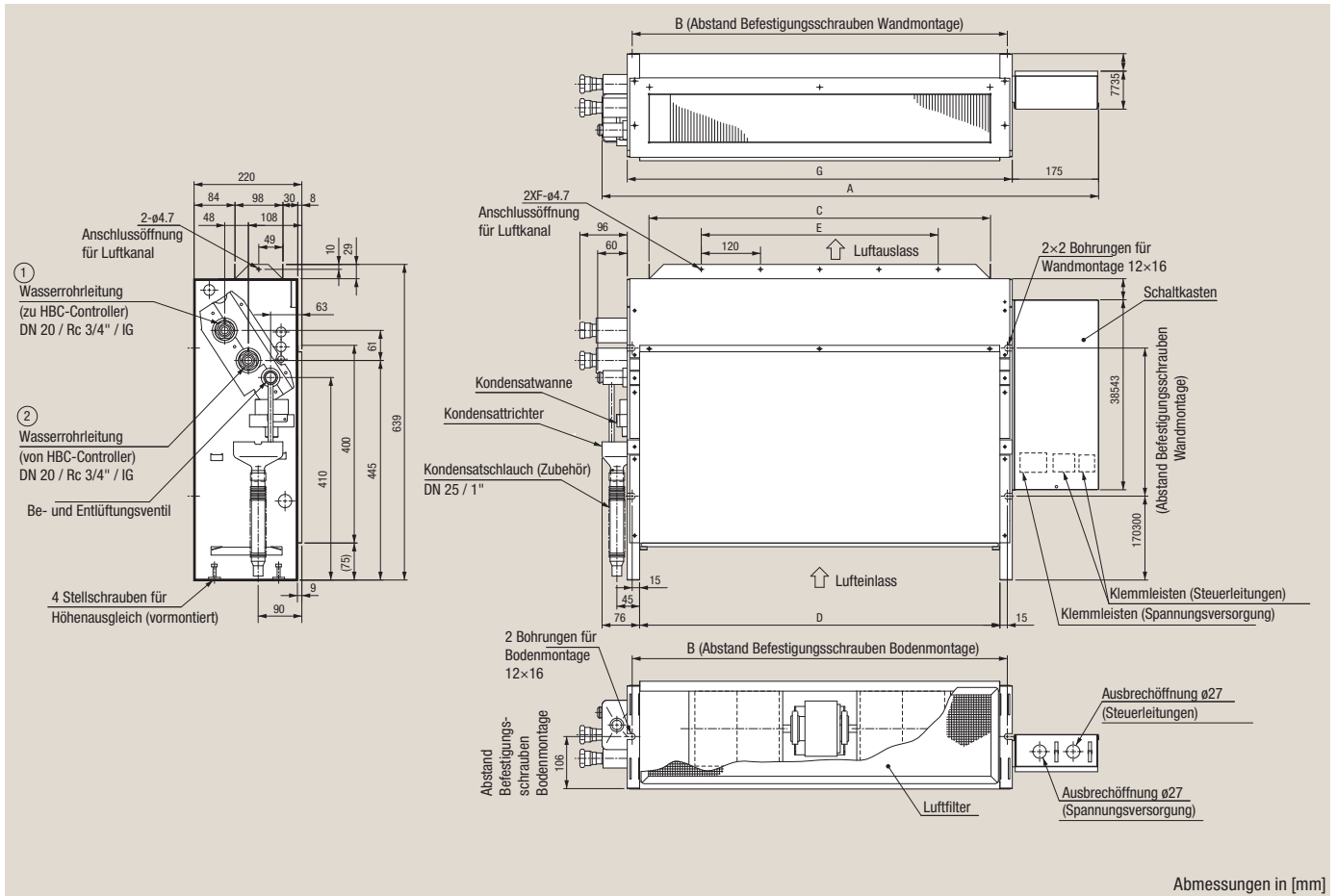
Abbildung 4.15 Abmessungen PFFY-WP20/25/32/40/50VLRMM-E
