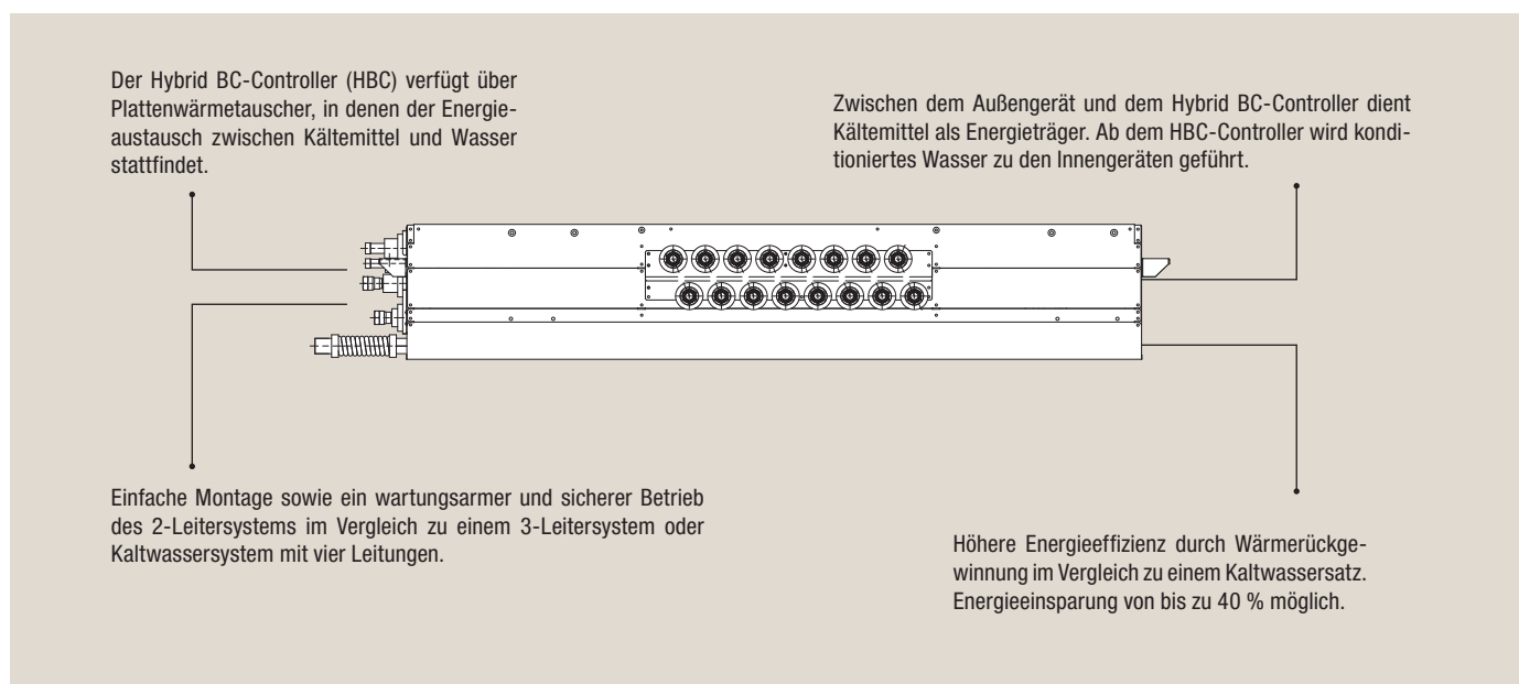
Abbildung 1.1 HBC-Controller
