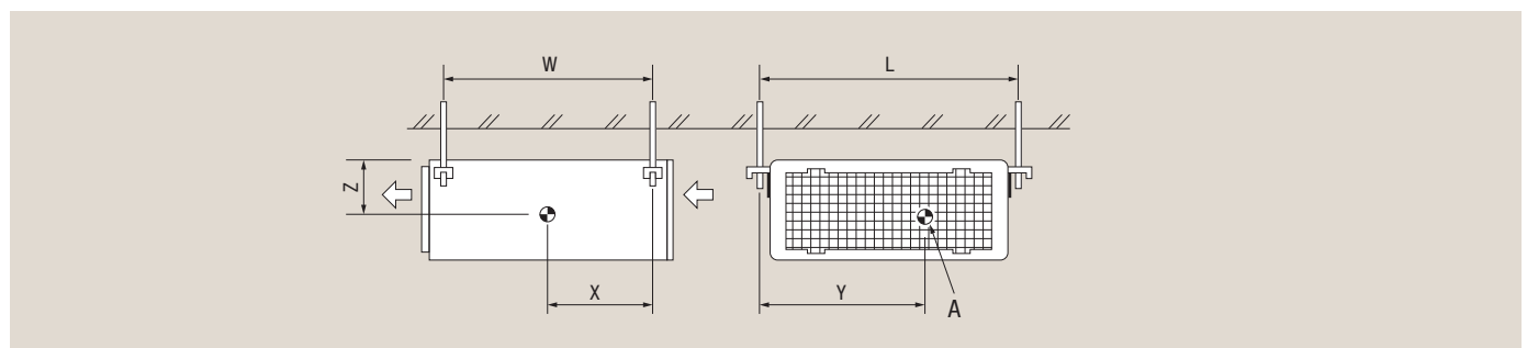
Abbildung 4.14 Schwerpunkt PEFY-WP20/25/32/40/50VMA-E
