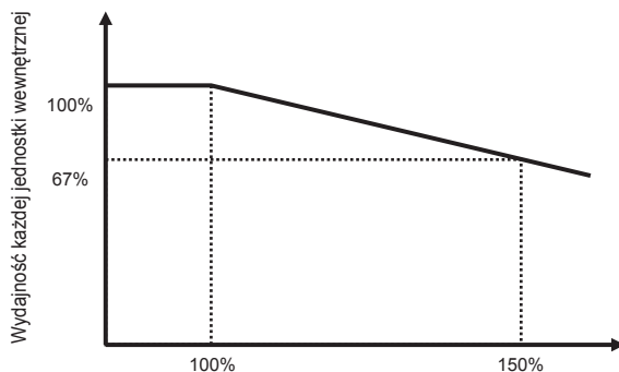
Stosunek łącznej wydajności jednostek wewnętrznych do wydajności jednostki zewnętrznej
