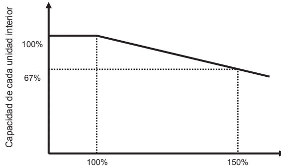
Relación entre la capacidad total de las unidades interiores y la capacidad de las unidades exteriores
