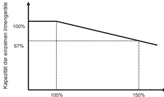
Verhältnis der Kapazität der Gesamtzahl Innengeräte zur Kapazität des Außengeräts Betriebsverhalten, wenn die Gesamtkapazität der verwendeten Innengeräte über der Kapazität des Außengeräts liegt.
