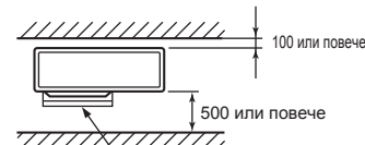
Насочващо струята устройство (MAC-856SG)
