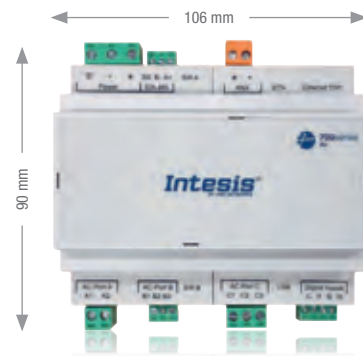
ME-AC-MBS-KNX-HA Schnittstelle
